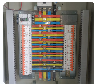
Tủ điện Electrical cabinets
